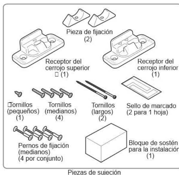
Piezas de sujeción
